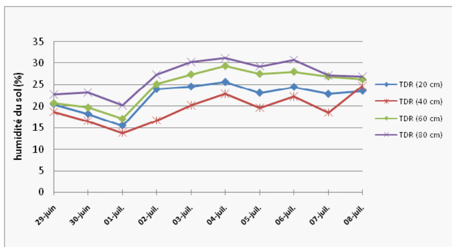
Figure 03: Variation du stock en eau du sol pour le système d’irrigation localisé à 20, 40,60 et 80 cm de profondeur pour la période estivale
