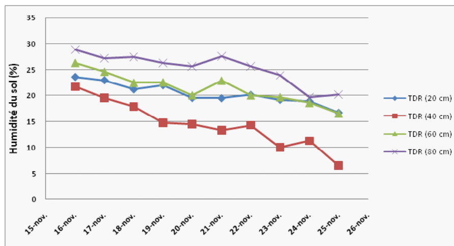
Figure 04: Variation du stock en eau du sol pour le système d'irrigation localisé à 20, 40, 60 et 80 cm de profondeur pour la période automnale.
