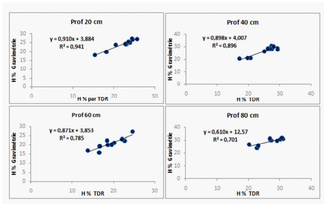
Figure 08 : Comparaison des stocks d'eau moyens sur les quatre niveaux de profondeur entre les mesures TDR et de gravimétrie Période estivale
