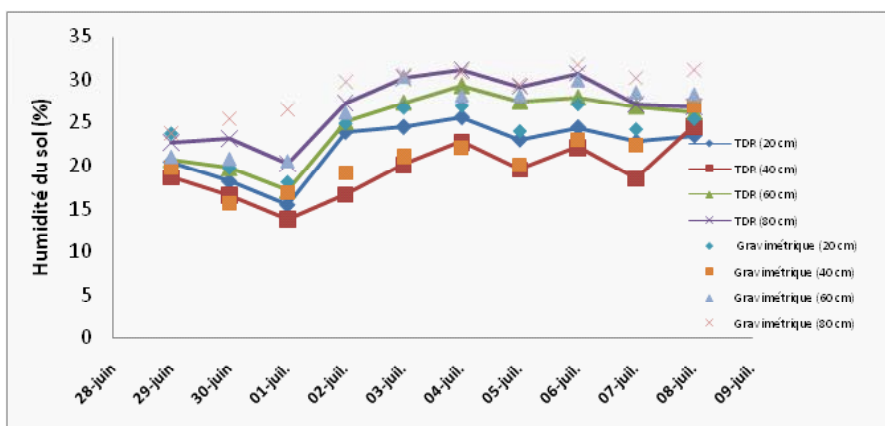
Figure 05: Evolution du stock d'eau selon les mesures TDR et les mesures gravimétriques pour les quatre couches d'un sol sableux pour la période estivale.
