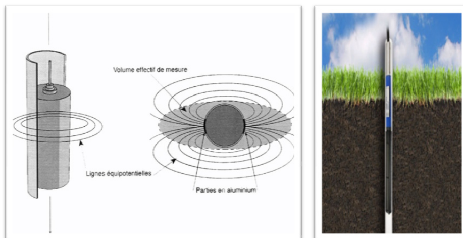
Figure 01 : Sonde tube TRIME et son volume de mesure
