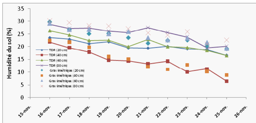
Figure 06: Evolution du stock d'eau selon les mesures TDR et les mesures gravimétriques pour les quatre couches d'un sol sableux pour la période automnale.
