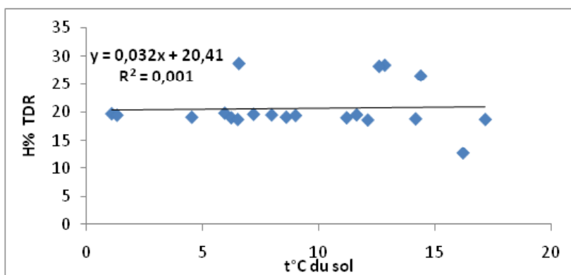
Figure 07 : Corrélation entre la température du sol et l'humidité de TDR
