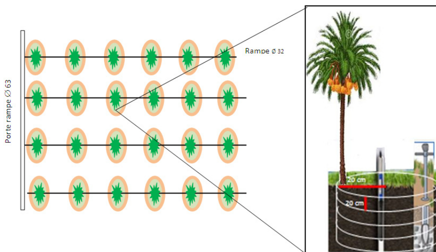
Figure 02 : Protocole de mesure de l’humidité du sol par la sonde TDR et la méthode gravimétrique.
