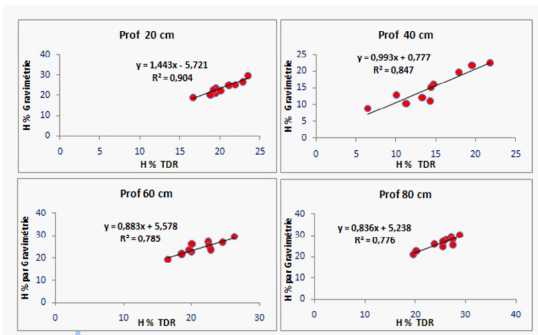
Figure 09: Comparaison des stocks d'eau moyens sur les quatre niveaux de profondeur entre les mesures TDR et de gravimétrie Période automnale
